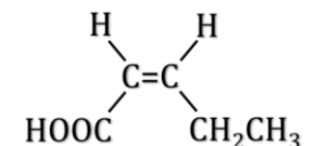
ácido cis-2-pentenoico
