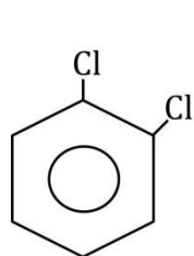
1,2-diclorobenceno
