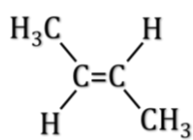
trans-2-buteno
