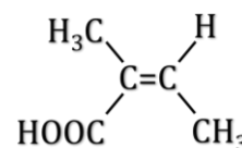
ácido trans-2-metil-2-butenico
