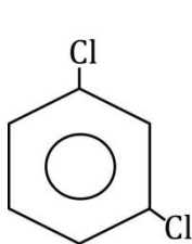
1,3-diclorobenceno
