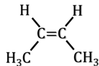
cis-2-buteno
