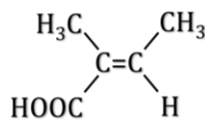
ácido cis-2-metil-2-butenico
