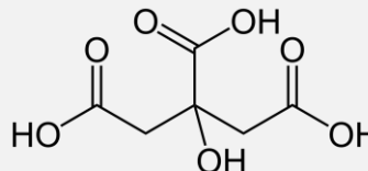
ácido cítrico
