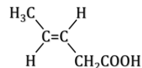
ácido trans-3-pentenoico
