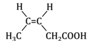
ácido cis-3-pentenoico
