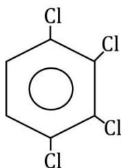
1,2,3,4-tetraclorobenceno
