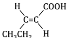
ácido trans-2-pentenoico
