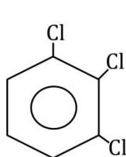
1,2,3-triclorobenceno
