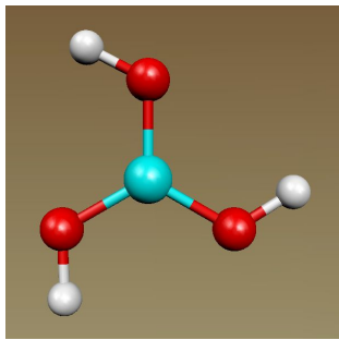
B(OH) 3 : C_{3h}
