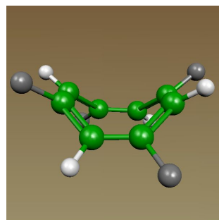
C 8 H 4 F 4 : S_4
