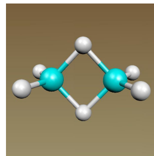
B 2 H 6 : D_{2h}
