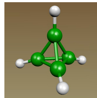
C 4 H 4 : T_d
