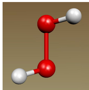
H 2 O 2 : C_2
