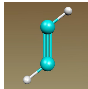
Si 2 H 2 : C_{2h}
