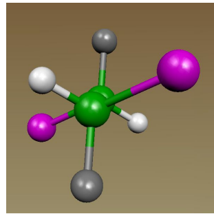
(CHFCI) 2 : C_i
