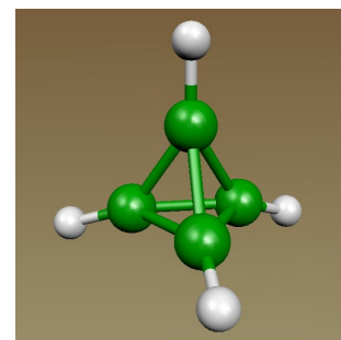
C 4 H 4 : ?
