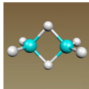
B 2 H 6 : ?
