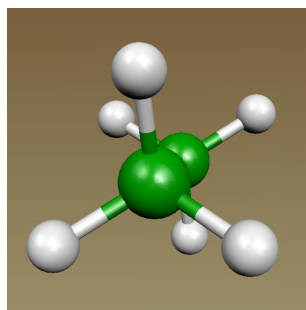
C 2 H 6 : ?
