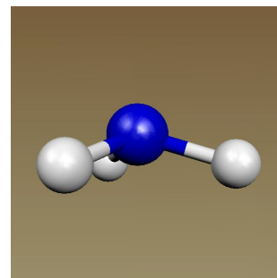
NH 3 : ?
