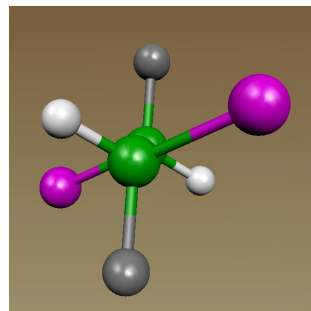
(CHFCI) 2 : ?
