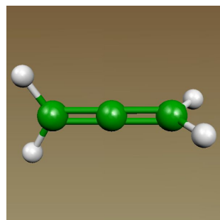
C 3 H 4 : ?
