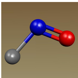
FNO: ?
