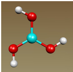
B(OH) 3 : ?
