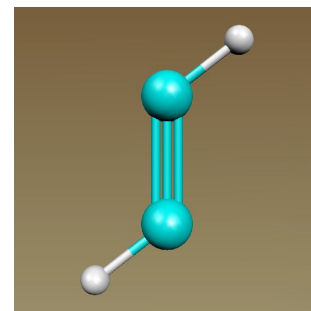
Si 2 H 2 : ?
