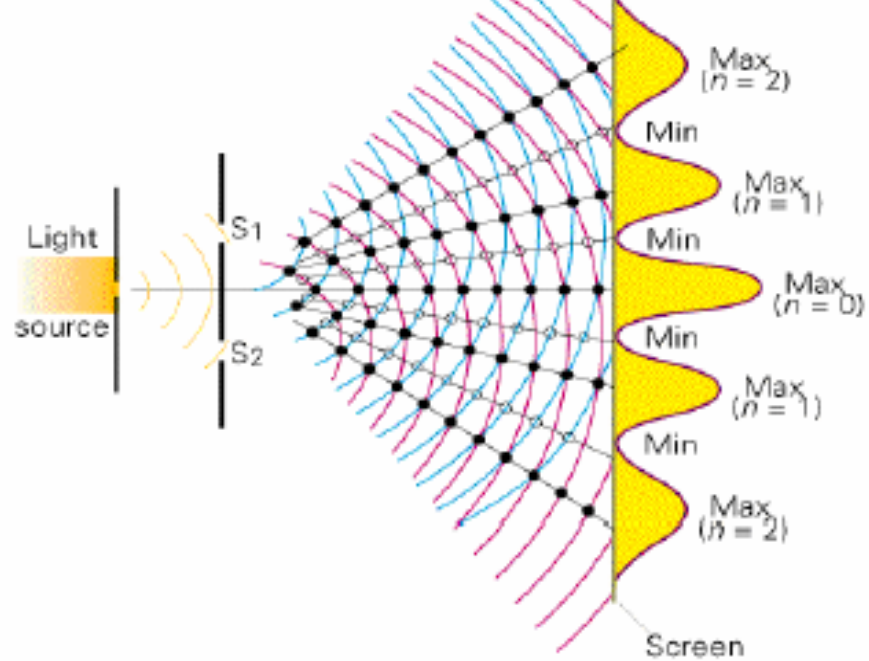
Interferencia destructiva
