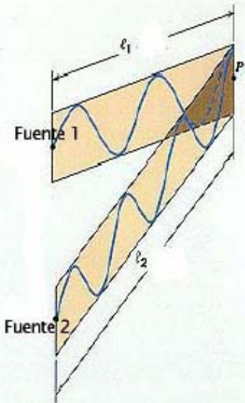
Interferencia constructiva
