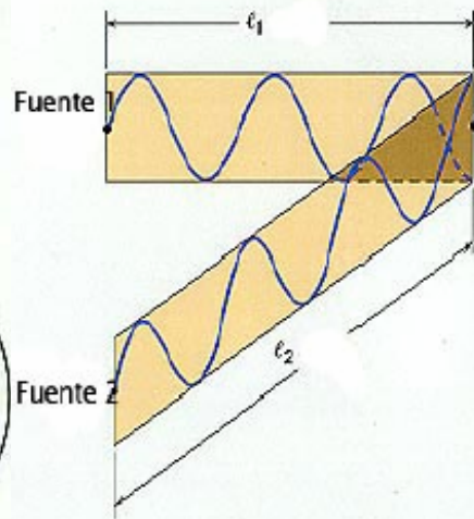
Interferencia destructiva
