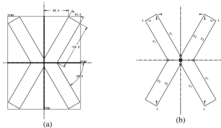
Figura 5: Modo esbozo de Pro/E: (a) ejemplo con una sección con cotas y (b) la misma sección con la intención de diseño (restricciones geométricas) capturada automáticamente por el administrador de intenciones de Pro/E
