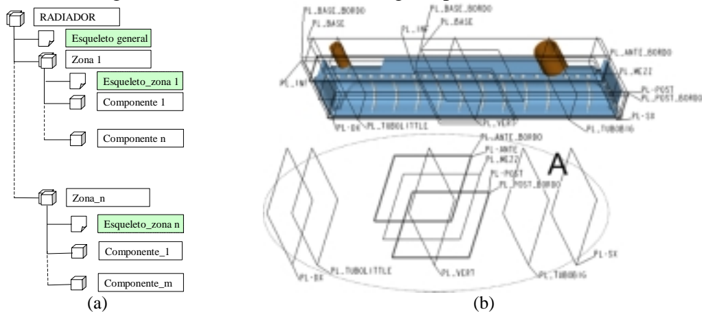
Figura 8: (a) Estructura del esqueleto de un radiador de automóvil dentro de la estructura del producto y (b) componente “depósito de salida” con geometría de detalle y su esqueleto
