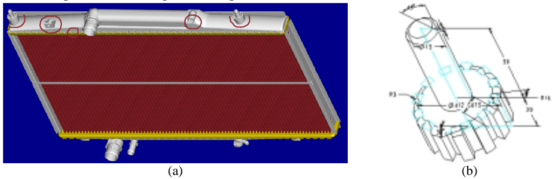
Figura 6: (a) Elementos de un radiador de automóvil candidatos a ser modelados como FDU (enmarcados en color rojo), y (b) creación de un modelo de pivote para anclaje mediante la función FDU de Pro/E
