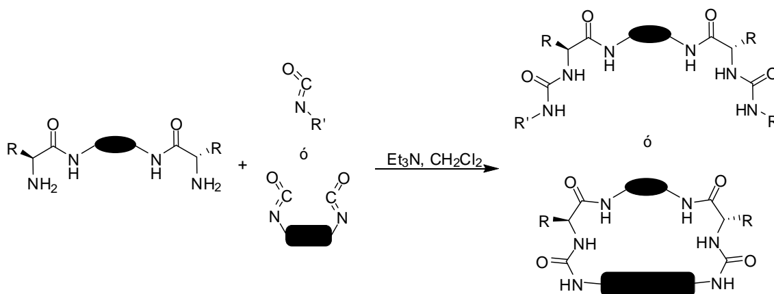
Esquema 1, Procedimiento sintético de la reacción entre un compuesto peptidomimético y un isocianato
